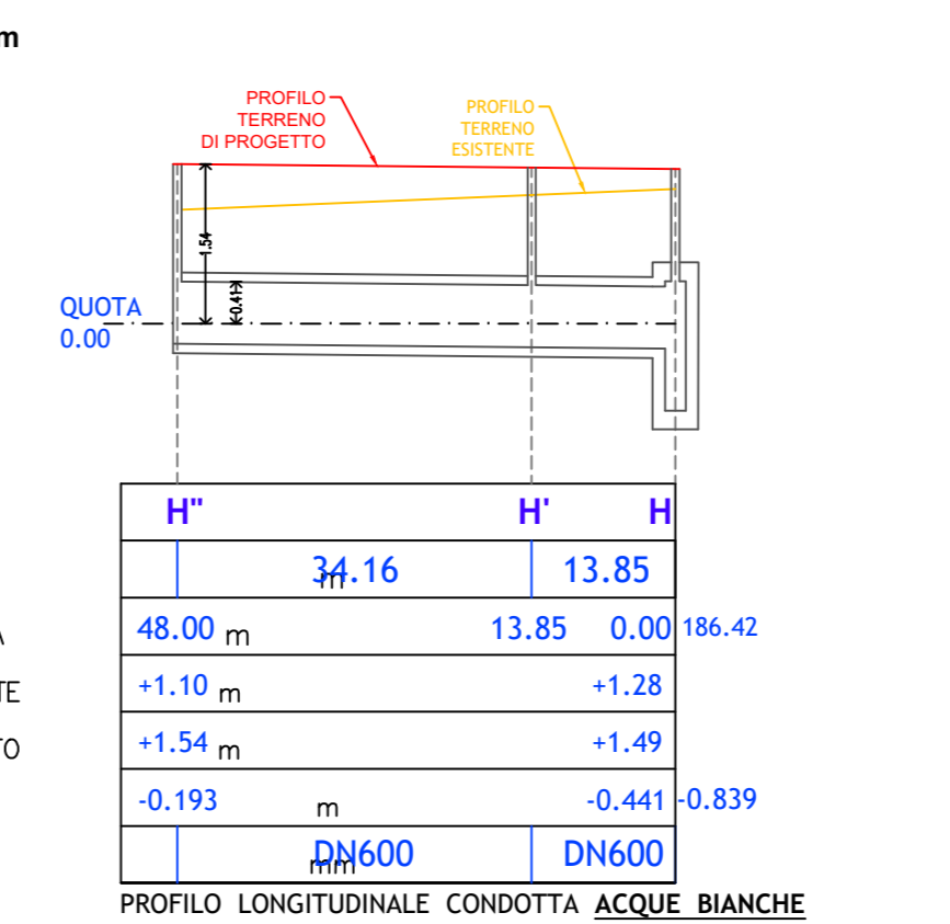
PROFLO LONGITUDINALE CONDOTTA ACQUE BIANCHE RAMO SECONDARIO H-H'
