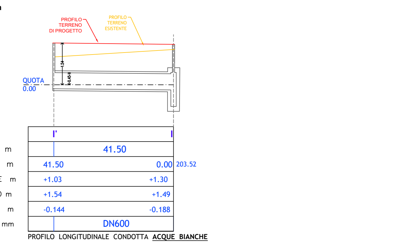
PROFLO LONGITUDINALE CONDOTTA ACQUE BIANCHE RAMO SECONDARIO I-I'
