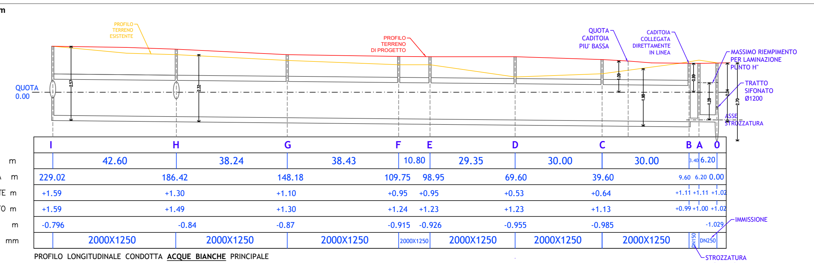
PROFLO LONGITUDINALE CONDOTTA ACQUE BIANCHE PRINCIPALE
