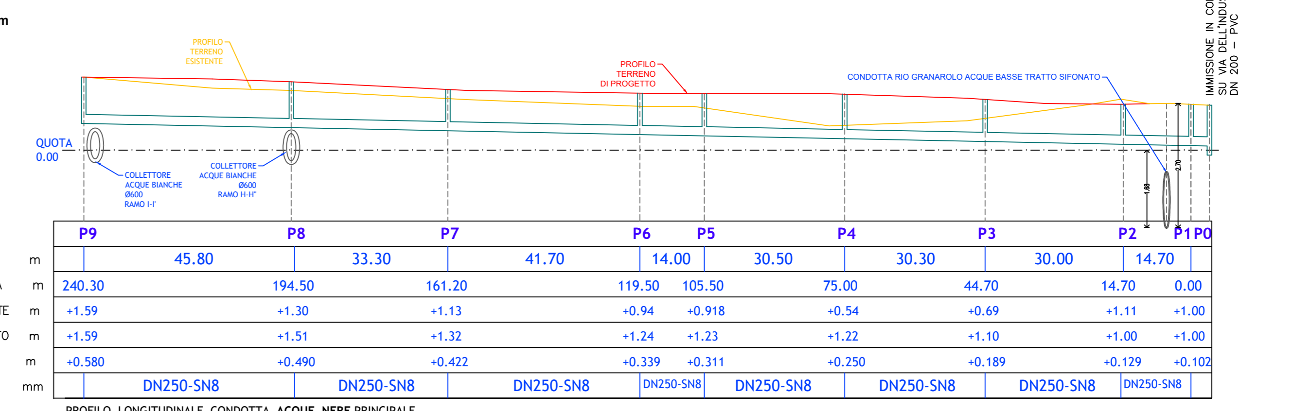
PROFLO LONGITUDINALE CONDOTTA ACQUE NERE PRINCIPALE
