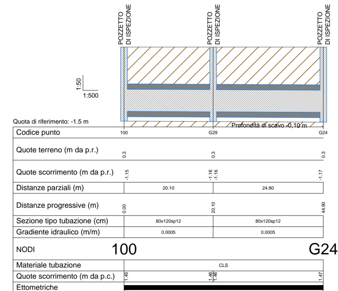
Profilo 100-G24
