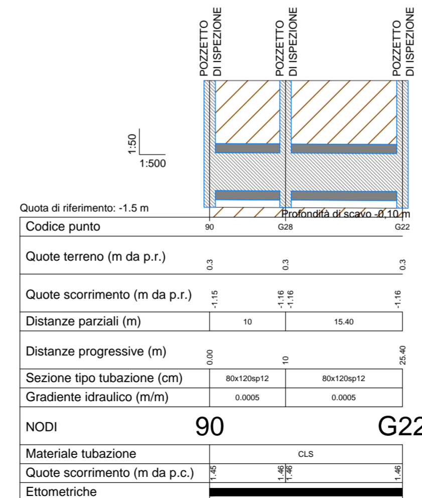
Profilo 90-G22
