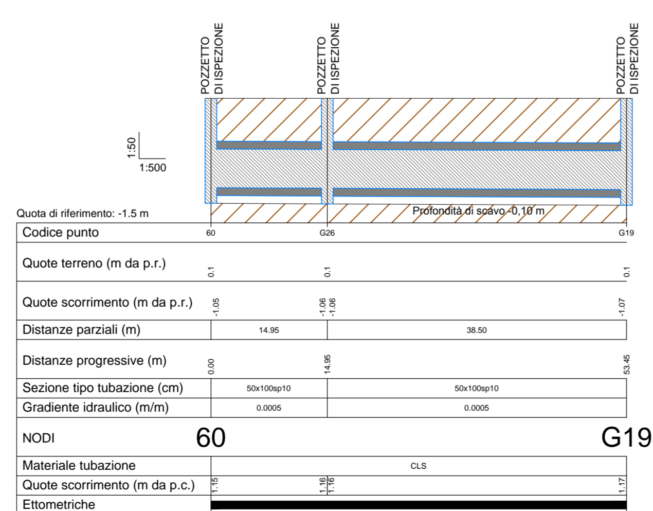
Profilo 60-G19
