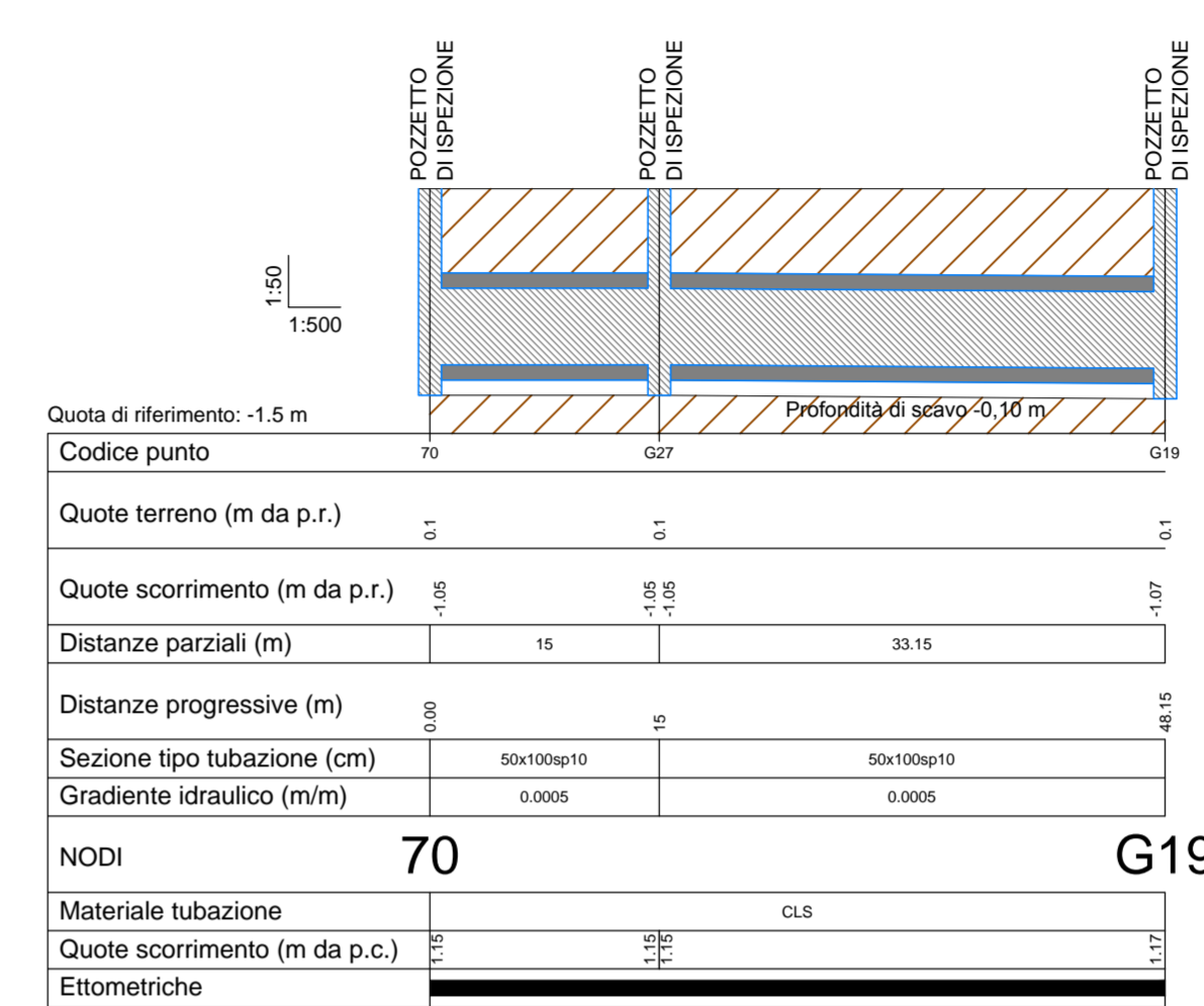
Profilo 70-G19
