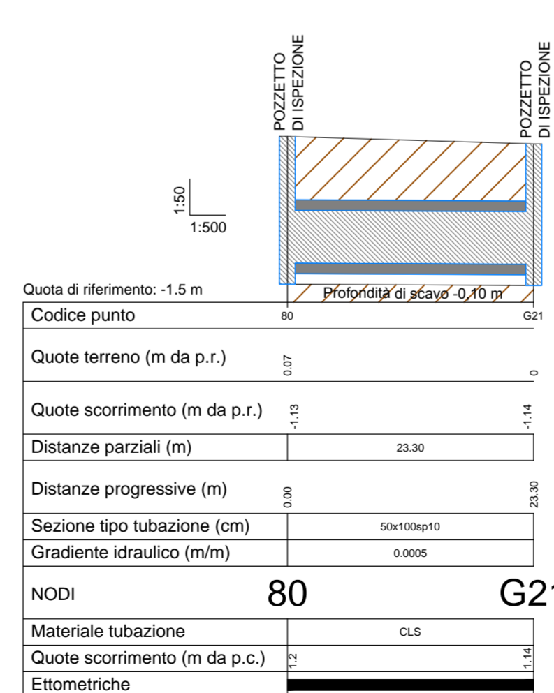
Profilo 80-G21
