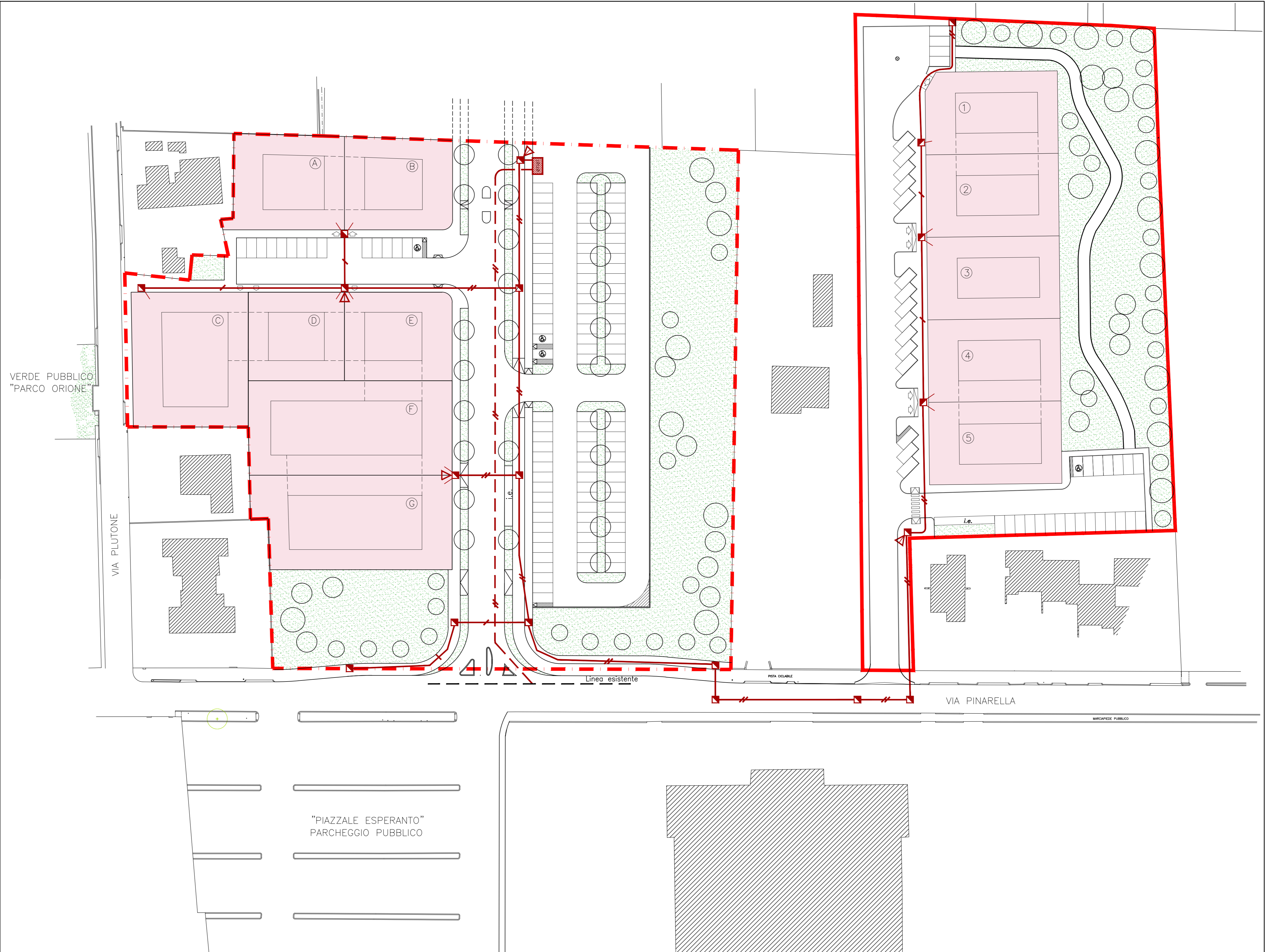
PLANIMETRIA SCALA 1:500
