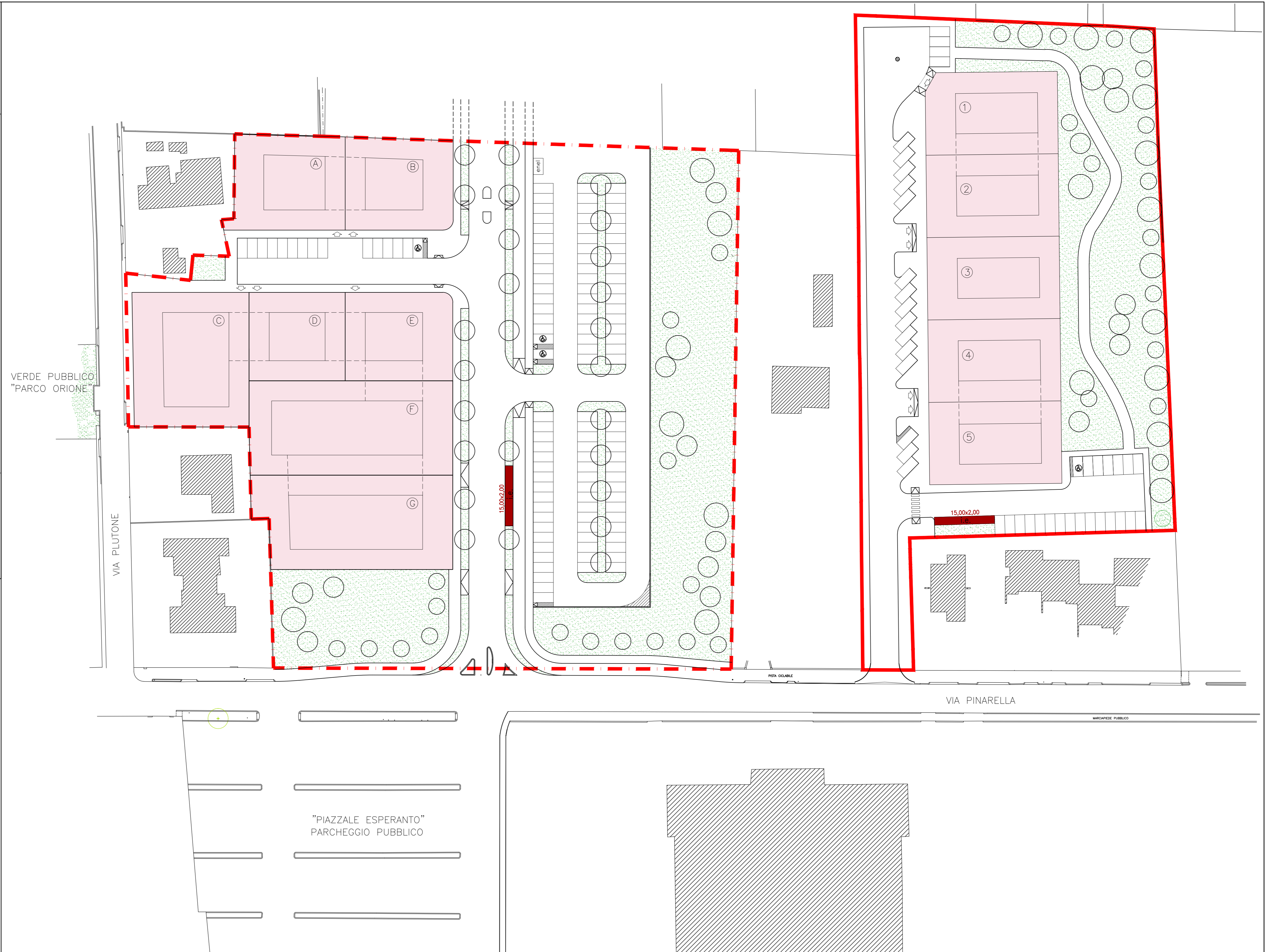
PLANIMETRIA SCALA 1:500
